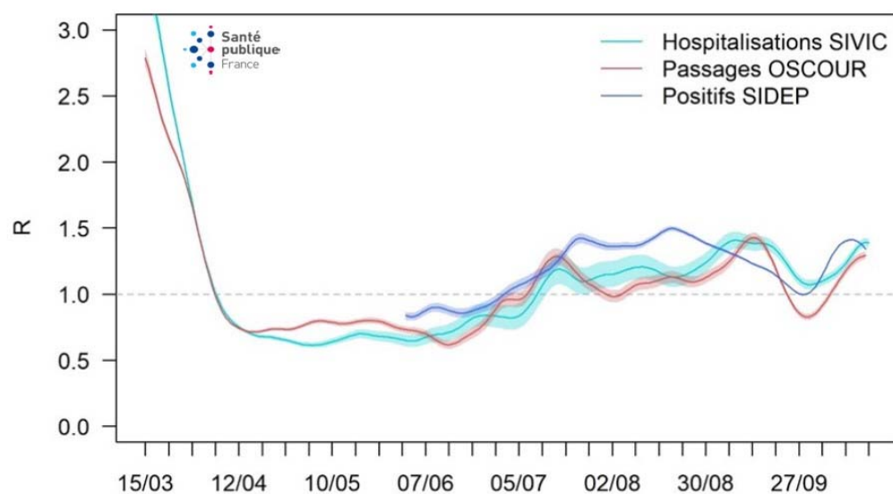
Figure 23. Trajectoire du nombre de reproduction effectif (R-effectif) à partir des tests PCR positifs au SARS-COV-2, des passages aux urgences avec suspicion de COVID-19 et des hospitalisations pour COVID-19 en France métropolitaine du 15 mars au 17 octobre 2020 (Sources : SI-DEP, OSCOUR® et SI-VIC)
